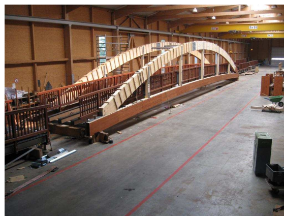
Bild 4: Fertigung
