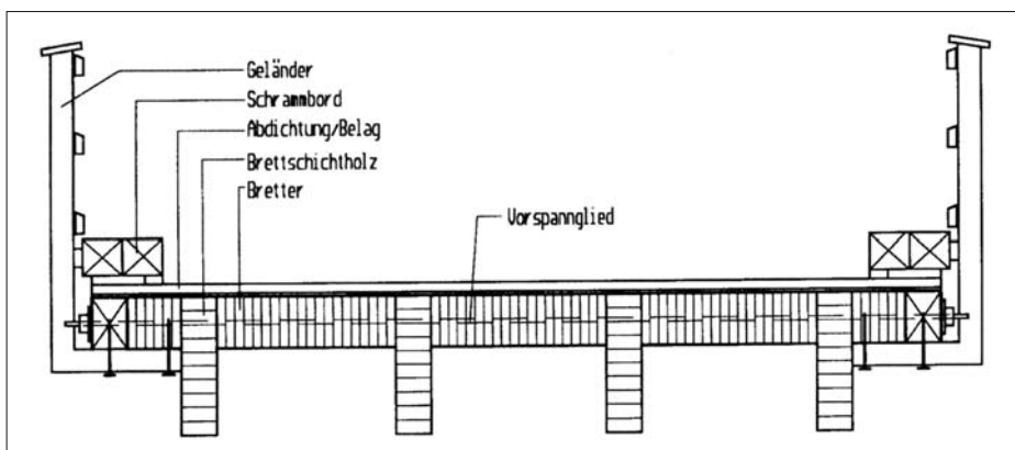
Bild 2.2 Quervorgespannte Holzplatte im Plattenbalken
