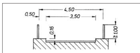
Bild 3.1 Profilm Maße für Brücken in einspurigen Wirtschaftswegen [DIN 1182]
