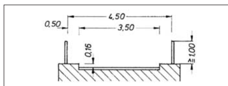
Bild 3.2 Profilm Maße für Brücken in einspurigen Wirtschaftswegen [DIN 1182]
