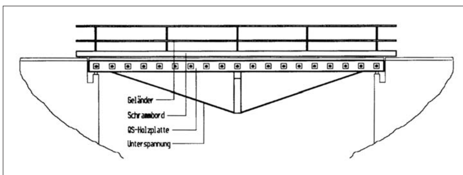
Bild 2.3 Einfach unterspannte Brücke mit QS-Holzplatte als Fahrbahn
