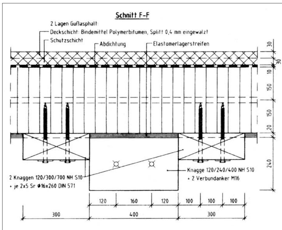
Bild 5.7 Knaagenausbildung
