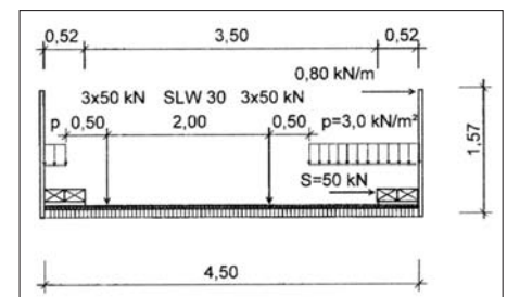
Bild 6.1 Lastbild (schematisch)
